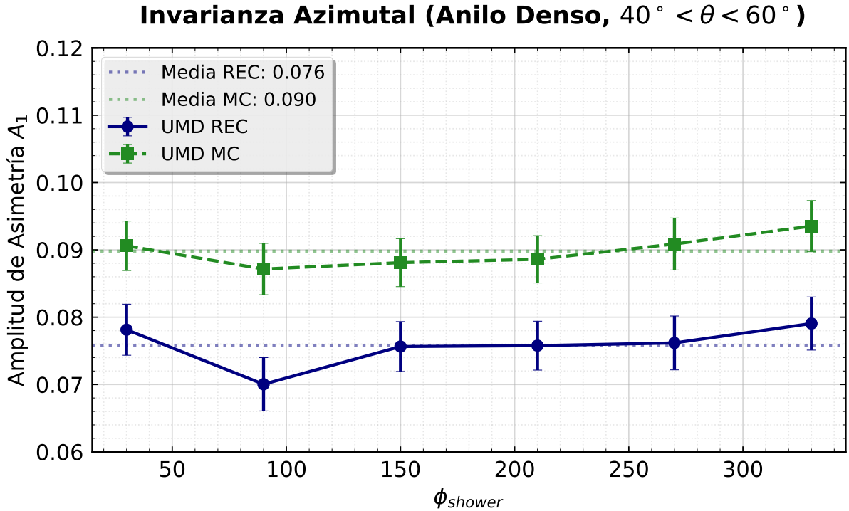
Figura 5.5: Amplitud A_1 en función del ángulo azimutal de la lluvia. Se observa la independencia del observable respecto a la dirección de arribo.
