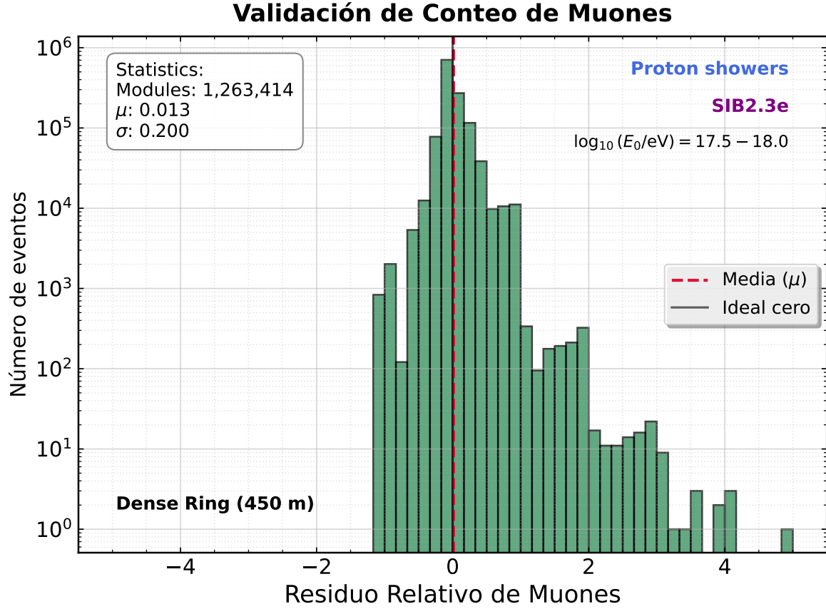
Figura 5.3: Resido Relativo de la reconstrucción de muones comparado con los inyectados para todas las lluvias de protones realizadas con el modelo Sibyll 2.3e en el anillo denso. Se obtuvo una media casi cero con una resolución pequeña en valor absoluto.
